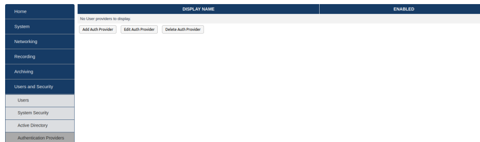
Fig. 7.42 Auth Providers
