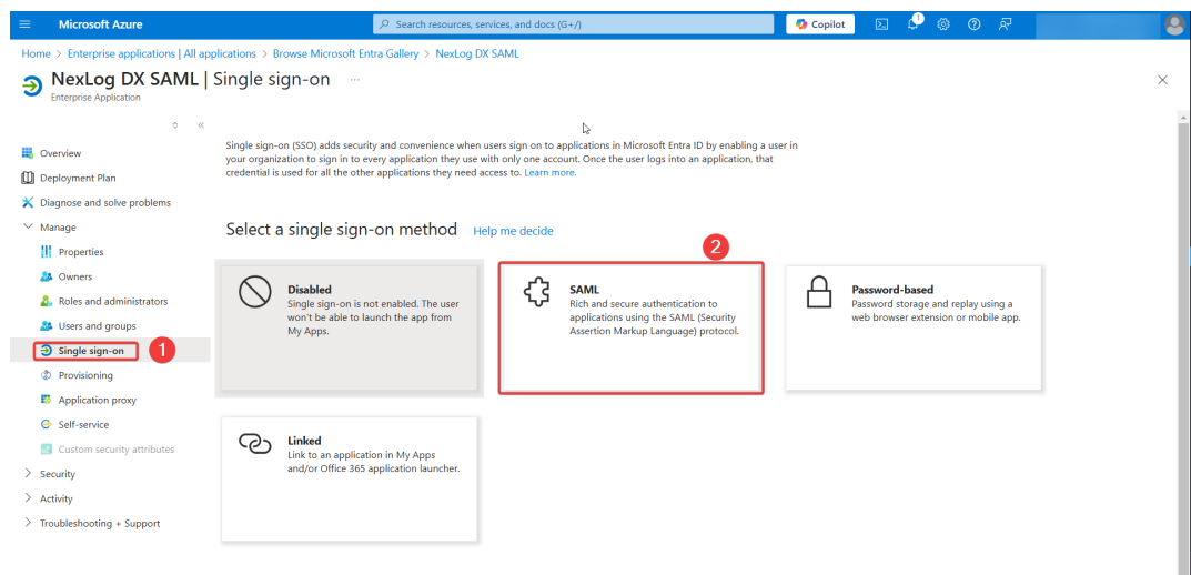
Fig. 7.27 Enable SAML
