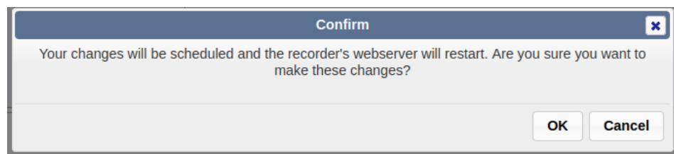
Fig. 7.45 Webserver Restart
