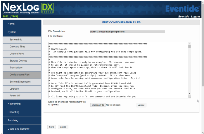
Fig. 7.27 SNMP Configure
