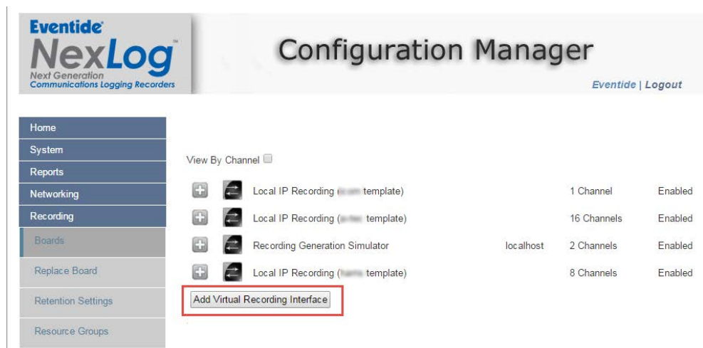
Fig. 6.103 Add Interface
