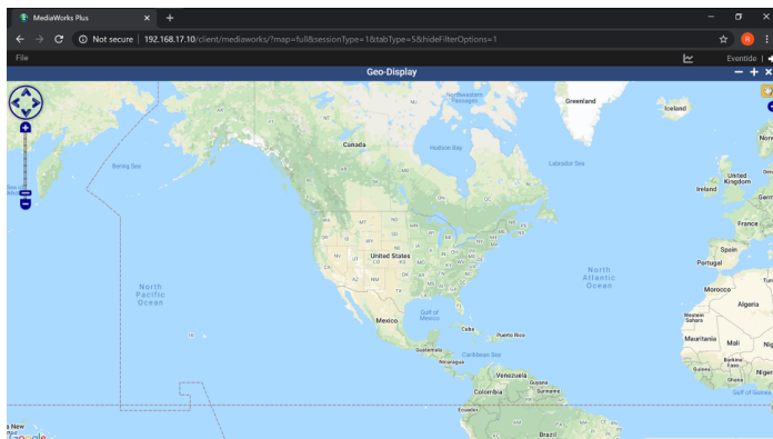
Fig. 17.9 Map
