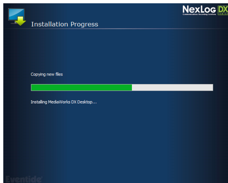
Fig. 15.1 Installer
