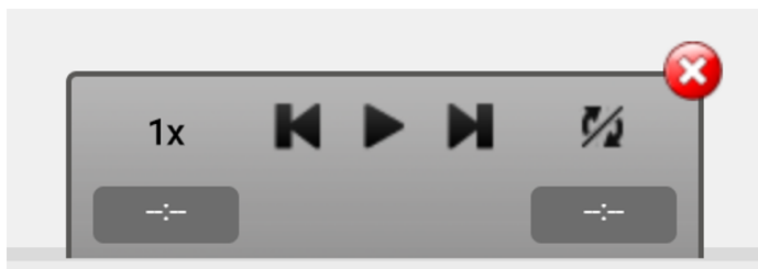
Fig. 17.4 Mini Transport
