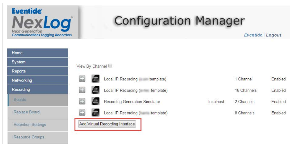
Fig. 6.124 Add Interface
