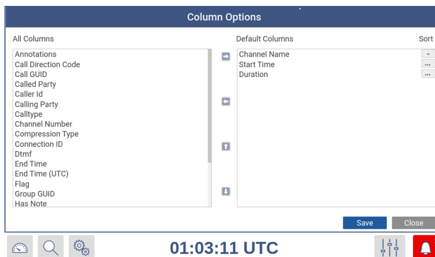
Fig. 6.21 Column Options
