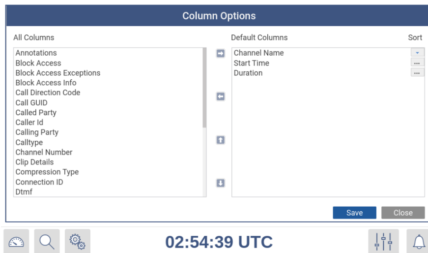
Fig. 6.20 Column Defaults
