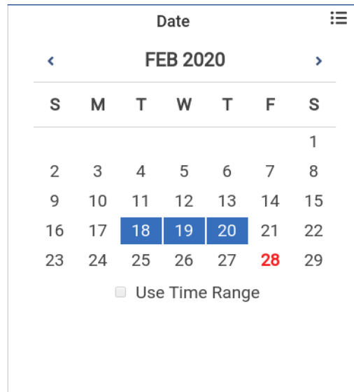
Fig. 6.17 Calendar
