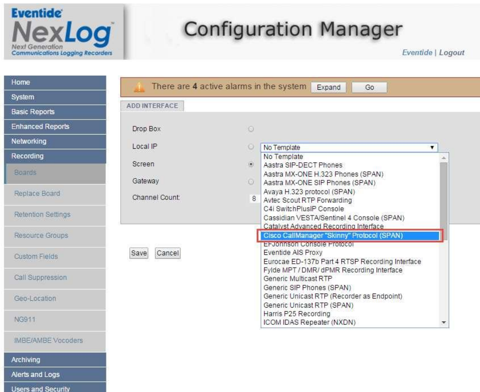
Fig. 6.60 Select Template
